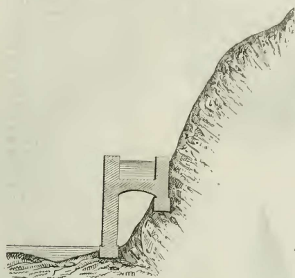
(Fig. 1. — Conduite d'eau le long des flancs des montagnes.)
